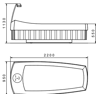
AquaThermoJet dimensions
