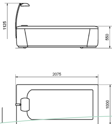
AquaThermoJet dimensions
